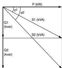
Fig. 1 : diagramme S
