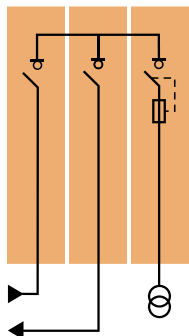
Exemple de tableau HTA type SM6 ou FluoKit avec 2 cellules interrupteurs de boucle et une cellule protection transformateur.
