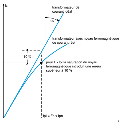
Courbe de saturation d'un noyau de transformateur de mesure et facteur de sécurité (Fs)
