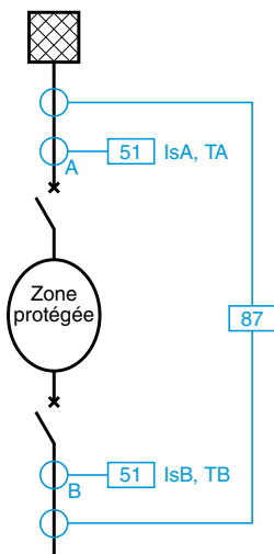
Sélectivités différentielle + chronométrique
