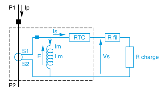
Schéma équivalent du circuit secondaire d'un TC
