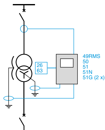
Transformateur faible puissance HT/HT
