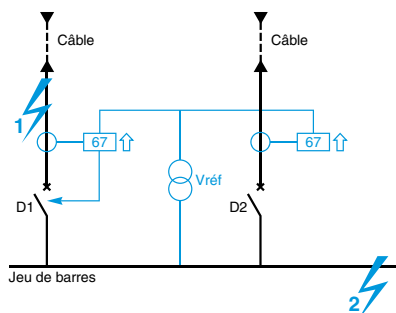
Protection directionnelle : exemple de deux arrivées en parallèle.
