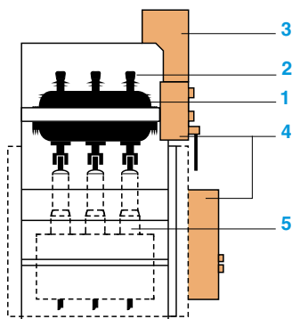
Cellule disjoncteur : exemple de LSC2A -PI (ancienne classification : compartimenté à appareil fixe ou débrochable)
