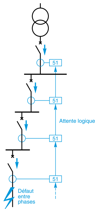
Principe de la sélectivité logique
