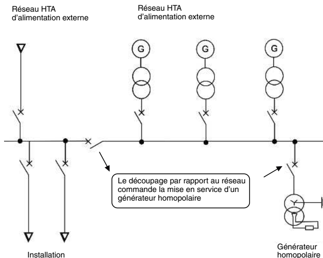
Schéma d'alimentation incluant des sources internes pouvant être couplées au réseau HTA
