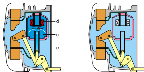
3 - Coupure d'arc
