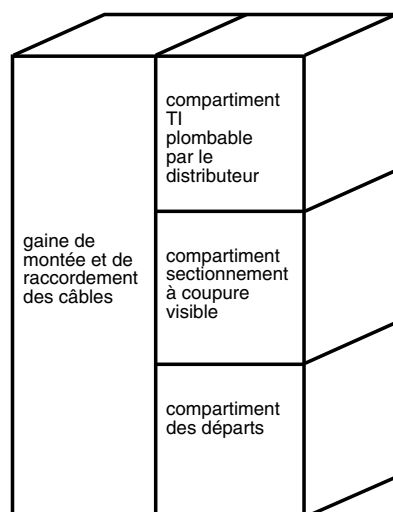
Compartiments du tableau BT
