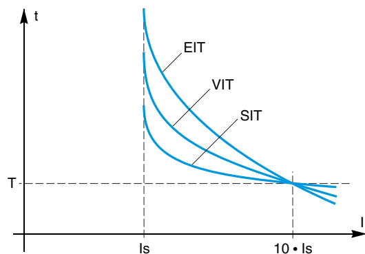
(3) Courbes CEI de déclenchement à temps dépendant
