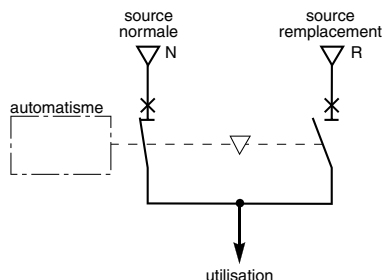
Inverseur de source
