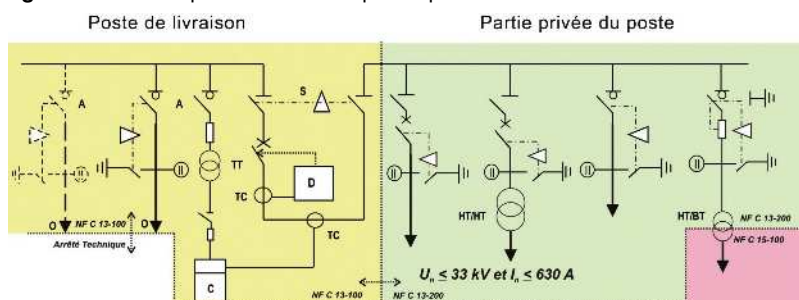
figure 13A – Exemple d'alimentation par un poste de livraison U \leq 33 kV et I_n \leq 630 A.
