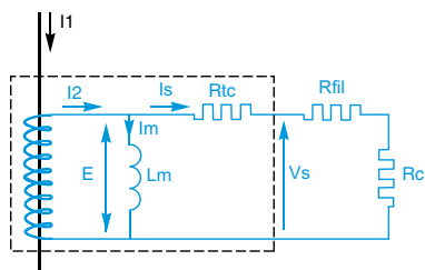
Schéma équivalent d'un transformateur de courant
