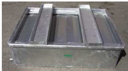
Exemple de bac d'extinction naturelle de l'offre Schneider Electric
