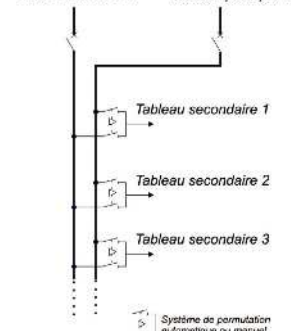
Fig. 31K - Double dérivation
