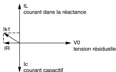
Diagramme vectoriel des courants lors du défaut terre
