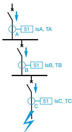
Réseau en antenne avec sélectivité chronométrique
