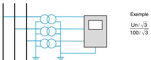
TT montés en étoile et exemple de rapport de transformation
