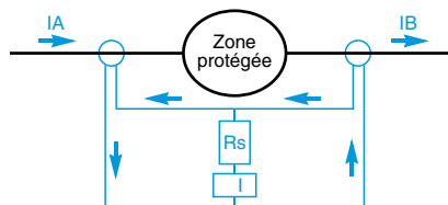
(3) schéma de protection différentielle à haute impédance.
