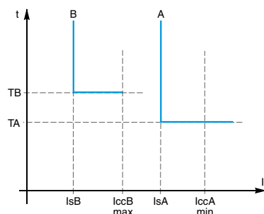
Courbes de sélectivité ampèremétrique
