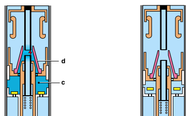
3 - Coupure d'arc
