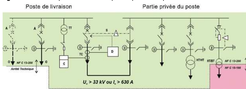
figure 13B – Exemple d'alimentation par un poste lorsque U > 33 kV ou I_n > 630 A.
