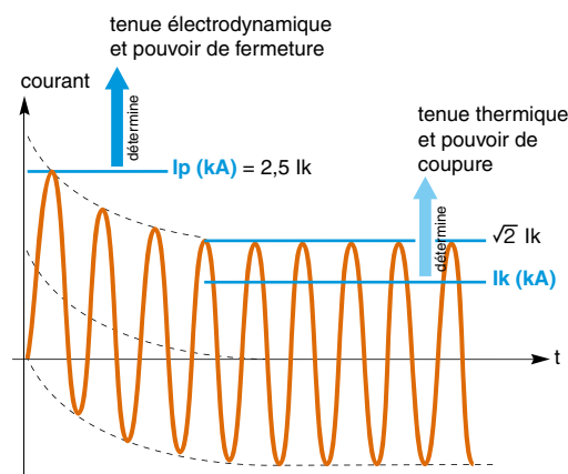
Courant de court-circuit normalisé
