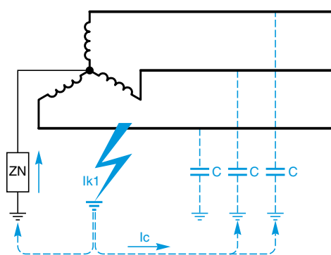
Schéma équivalent d'un réseau sur défaut à la terre. Les capacités C sont les capacités naturelles de fuite des câbles à la terre. Le courant I_c est le courant capacitif total du réseau se rebouclant à travers les phases saines du réseau.
