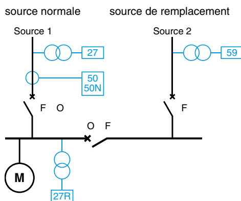
Transfert automatique de source
