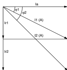
Fig. 2 : diagramme I
