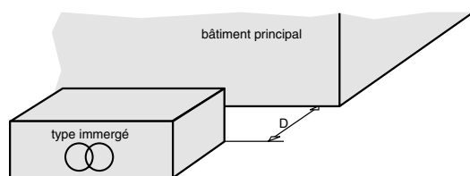
Poste d'extérieur avec transformateur immergé installé à une distance D d'un autre bâtiment
