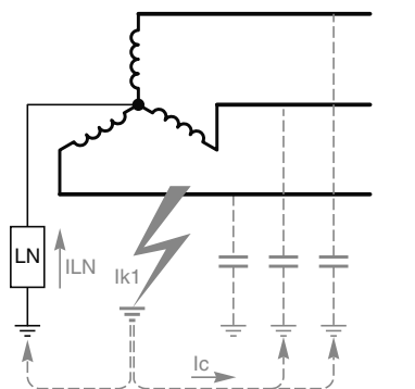
Réalisation de mise à la terre pour neutre accessible
