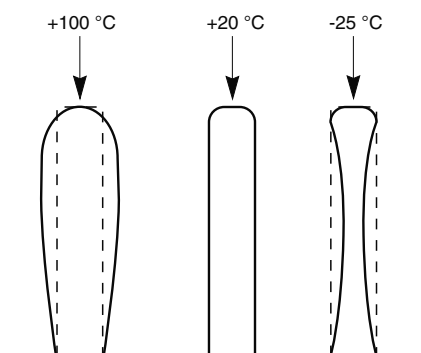
a - ERT : effet des variations température sur la déformations élastiques des ailettes
