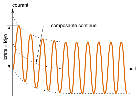
Forme du courant de court-circuit
