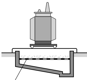
Dispositif d'extinction naturelle
