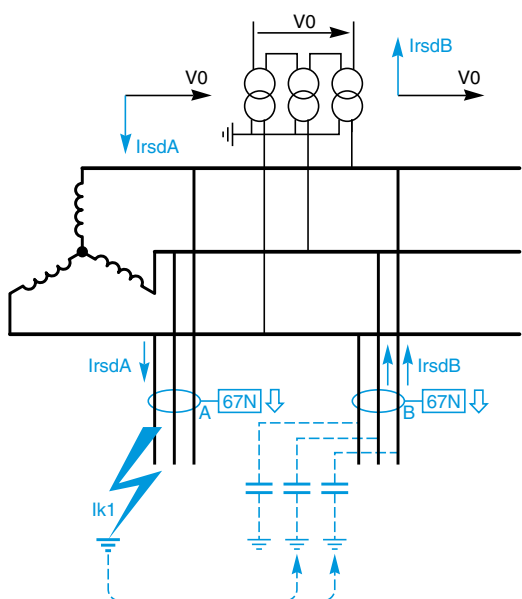
Détection par maximum de courant terre directionnelle
