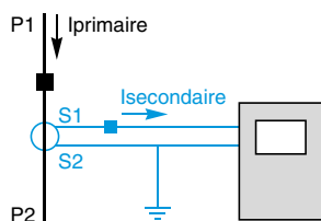
Transformateur de courant avec représentation des bornes.
