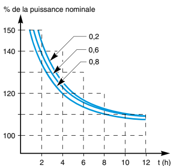
Transformateurs immergés
