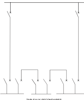
Fig. 31J - Boucle fermée
