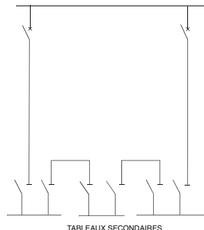
Fig. 31H - Boucle ouverte
