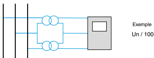
TT montés en V et exemple de rapport de transformation
