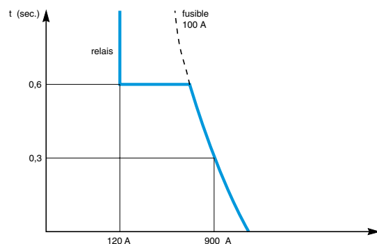
Figure 2 : protection transformateur par interrupteur-fusibles
