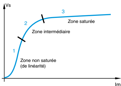
Courbe de magnétisation (d'excitation) d'un TC
