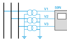
Fig. 2 : calcul de la tension résiduelle
