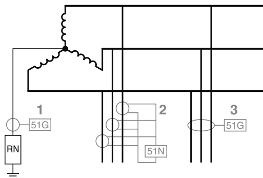
Fig. 5 : solutions de protection terre
