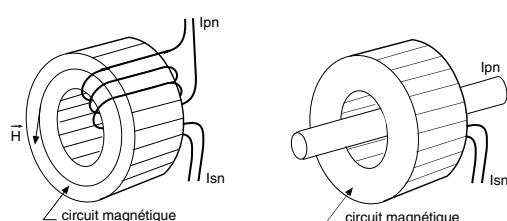
Transformateur de courant à primaire bobiné
