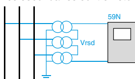
Fig. 1 : mesure directe de la tension résiduelle
