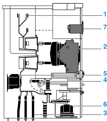
Cellule disjoncteur : exemple de LSC2B -PM (ancienne classification : blindé à disjoncteur débrochable)
