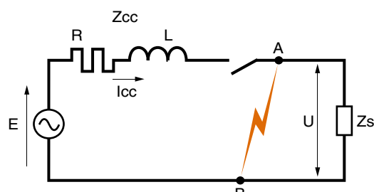
Éléments déterminant un courant de court-circuit
