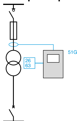
Transformateur faible puissance HT/BT protection fusible
