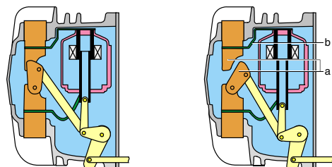
1 - Disjoncteur fermé
