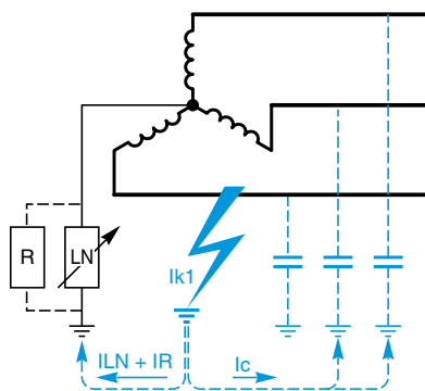
Défaut à la terre dans un réseau avec réactance de compensation à la terre
