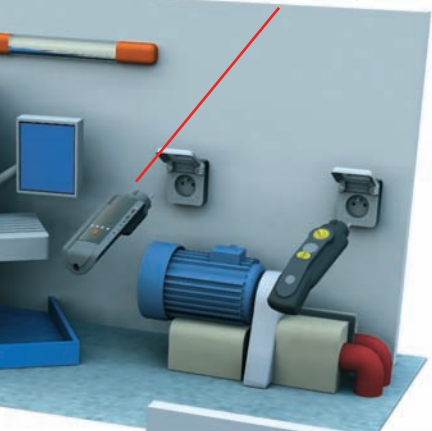
Contrôle de différentiels sur prise 2P+T avec le Catex™ NG (Réf. DT-170).
